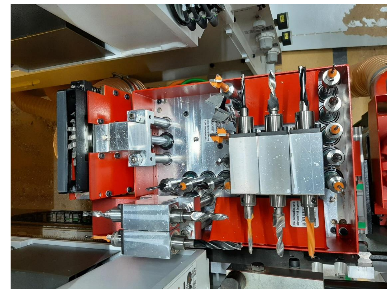
Bohrkopf
